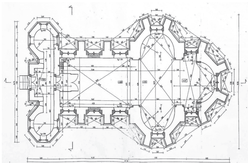
Fig. 2 – Biserica Mănăstirii Florești. Plan și relevu. Scara 1/100. Autor: arhitect Radu Pană, 1991.
