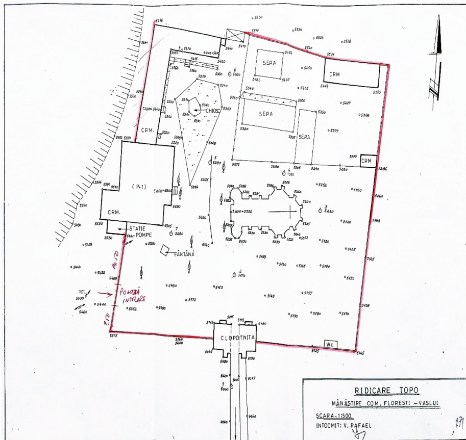
Fig. 3 – Mănăstirea Florești. Plan și ridicare topografică. Scara 1/500. Autor: arhitect V. Rafael, 1991.
