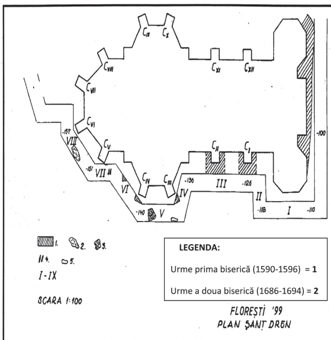
Fig. 1 – Biserica Mănăstirii Florești. Plan, etape evoluție și șant dren. Apud C. Asăvoaie, L. Chiriac, Noi date istorico-arheologice privind Mănăstirea Florești, județul Vaslui , în „Acta Moldaviae Meridionalis”, XXI, 1999-2000, 2001, p. 68.
